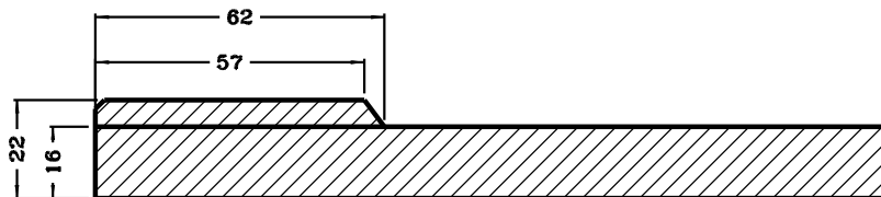
DOORSNEDE DEUR
