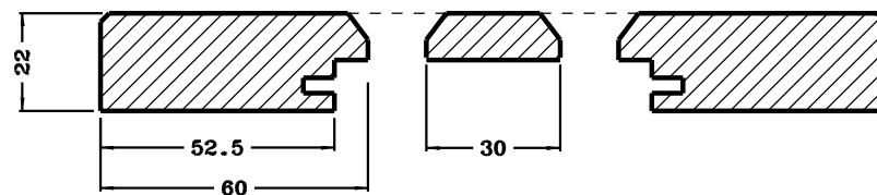
DOORSNEDE RAAMDEUR/SPIJLRAAMDEUR
